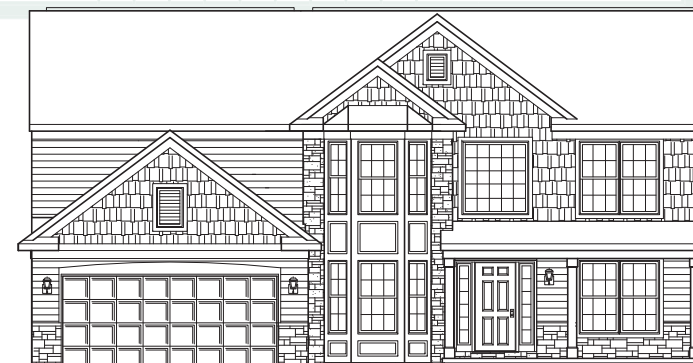
Elevation "H"
